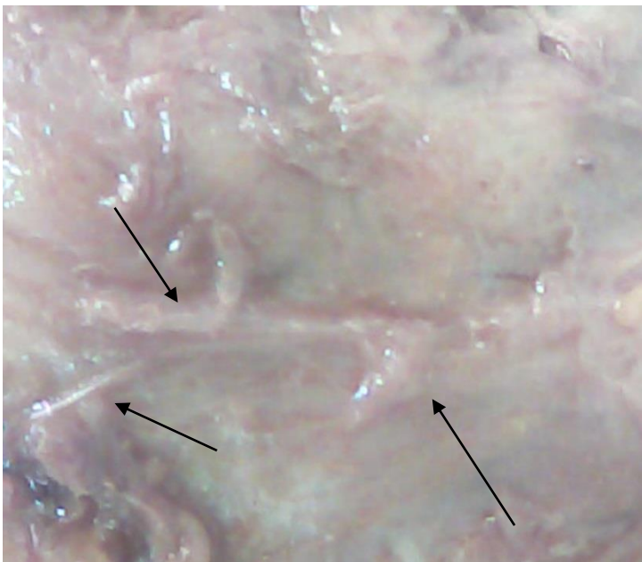
სურათი 37. კიბოვანი პროსტატის ინფრაწითელი გამოსახულება უკუგაბნეულ სხივებში. ისრებით ნაჩვენებია პროსტატის ზედაპირის არაჰომოგენურობა.
