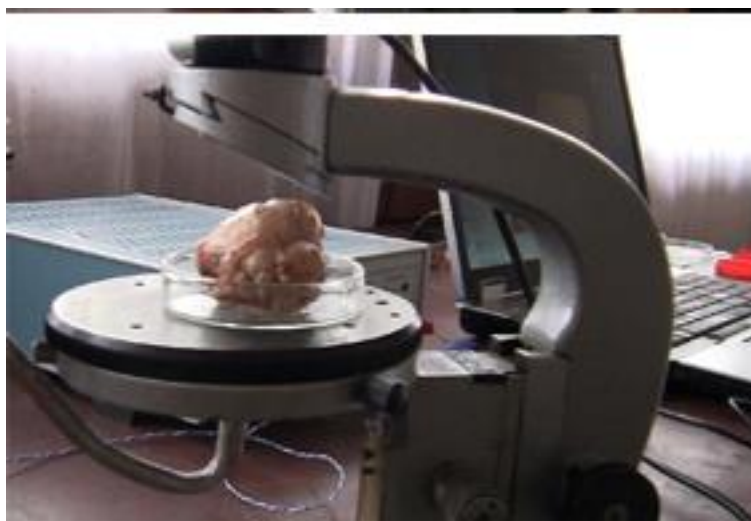
სურათი 8. ინფრაწითელი სხივები, რომლებიც გამოდიან ფოტოდიოდიდან, განჟოლავენ მთლიან პროსტატას და ხვდებიან CCD კამერაში.
