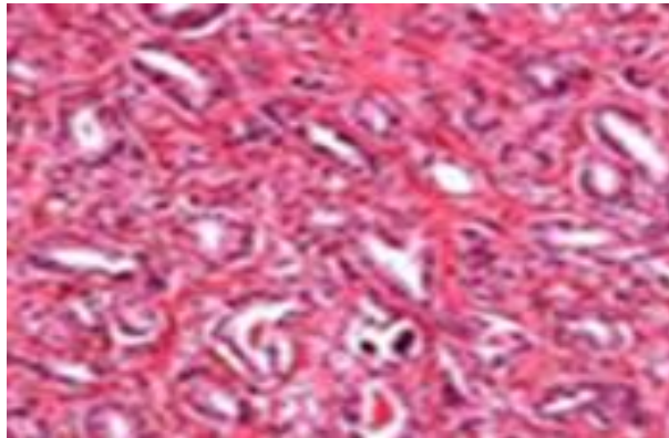
სურათი 27. კიბოვანი წარმონაქმნი შედგება კომპლექსური ბადისებური ურთიერთ შეზრდილი სტრუქტურებისაგან. სტრომასთან შეზრდა არ დაიმზირება.
