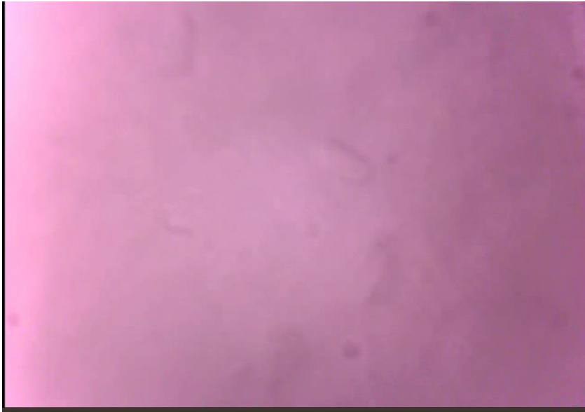
სურათი 51. დამუშავებული ხელსაწყოთა საშუალებით მიღებული არაკიბოვანი პროსტატის ინფრაწითელი გამოსახულება. გამოსახულების განათებულიობა ჰომოგენურია, რადგან არ შეიცავს კიბოვან წარმონაქმნებს.
