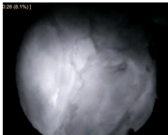
სურათი 18. პროსტატის ინფრაწითელი გამოსახულება. ფოტოდიოდის გამოსხივებული ენერგია არის 90 მვატ/სტერადიანზე. ამ ფოტოდიოდის გამოსხივების კუთხე 90° ტოლია. გამოსახულება დაიმზირება რექტუმის მხარედან.
